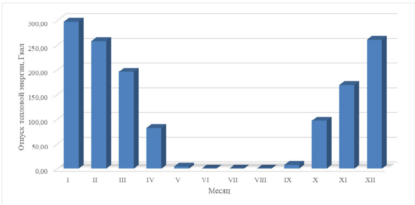
Рисунок 1.6 – Оптимальный температурный график отпуски тепловой энергии по котельной «УПК»
