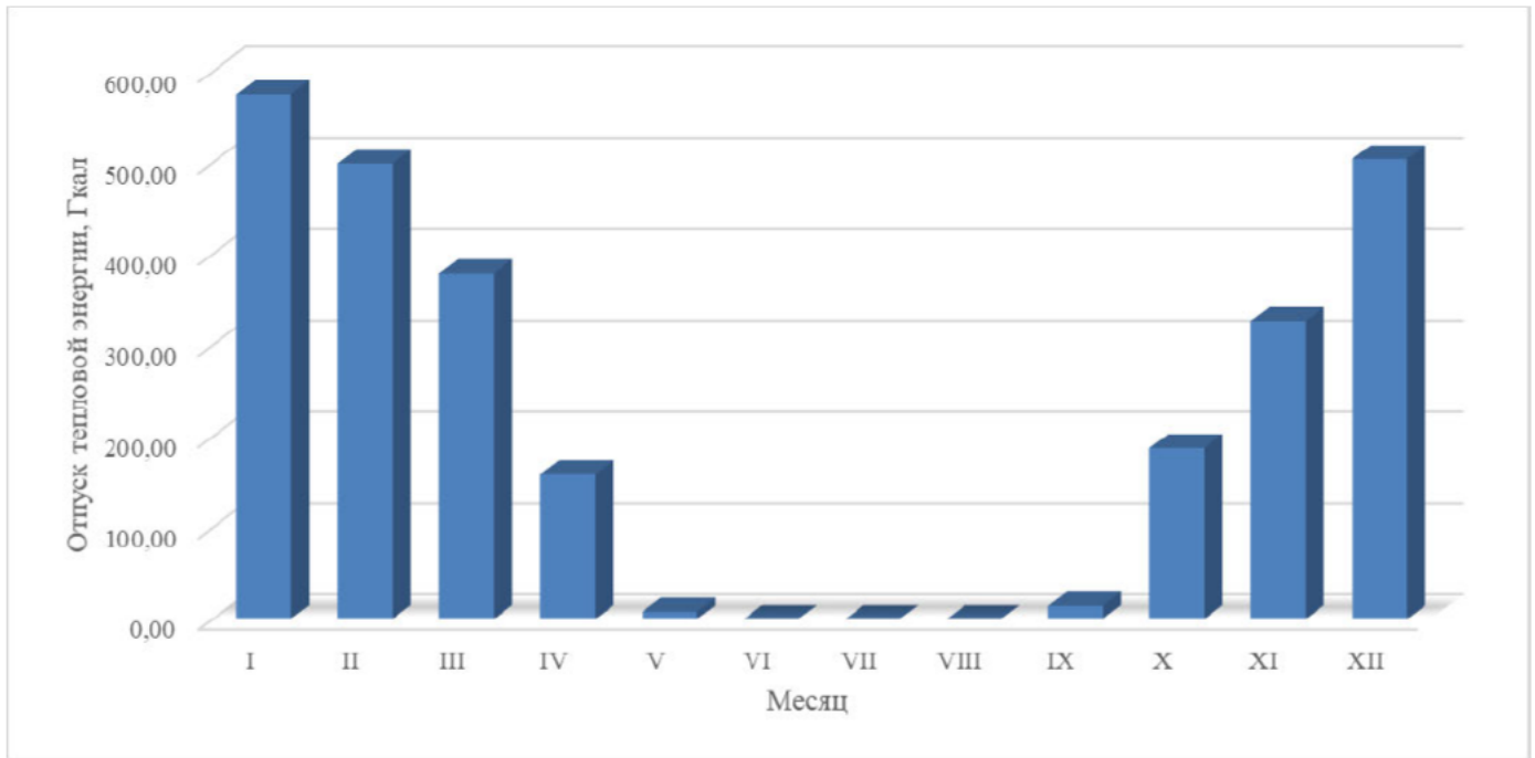
Рисунок 1.5 – Оптимальный температурный график отпуски тепловой энергии по котельной «Больница»
