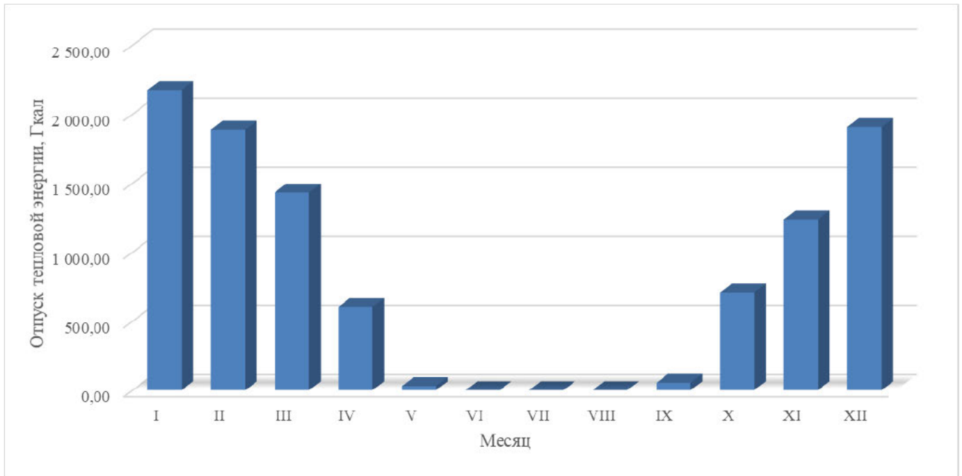
Рисунок 1.3 – Оптимальный температурный график отпуски тепловой энергии по котельной «Микрорайон»
