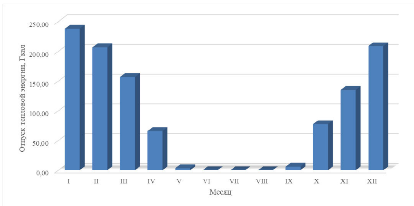
Рисунок 1.3 – Оптимальный температурный график отпуски тепловой энергии
