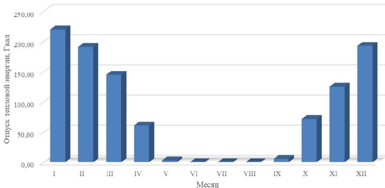
Рисунок 1.3 – Оптимальный температурный график отпуски тепловой энергии
