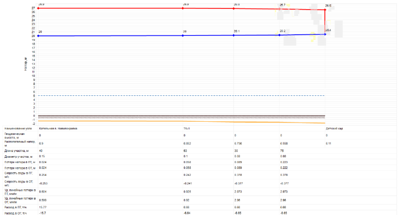
Рисунок 2.4 – Пьезометрический график работы котельной п. Новопокровка
