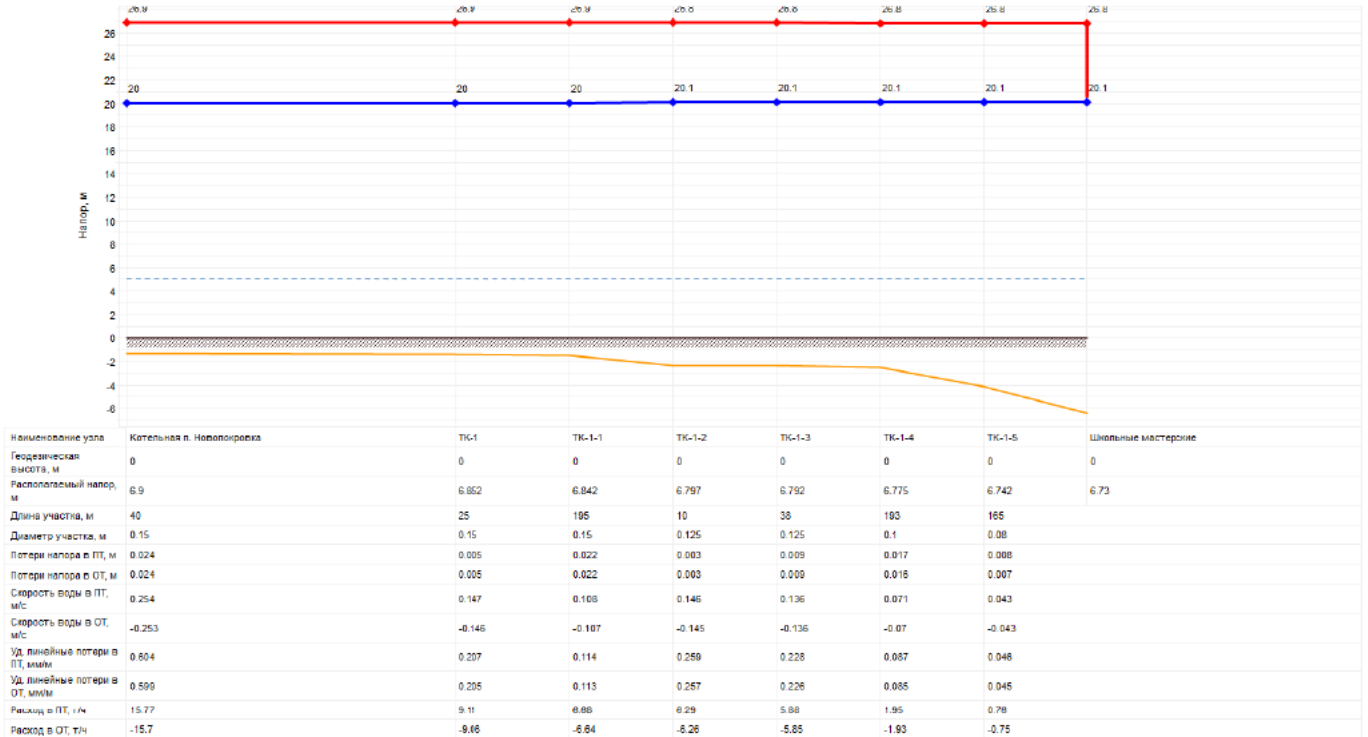
Рисунок 2.5 – Пьезометрический график работы котельной п. Новопокровка
