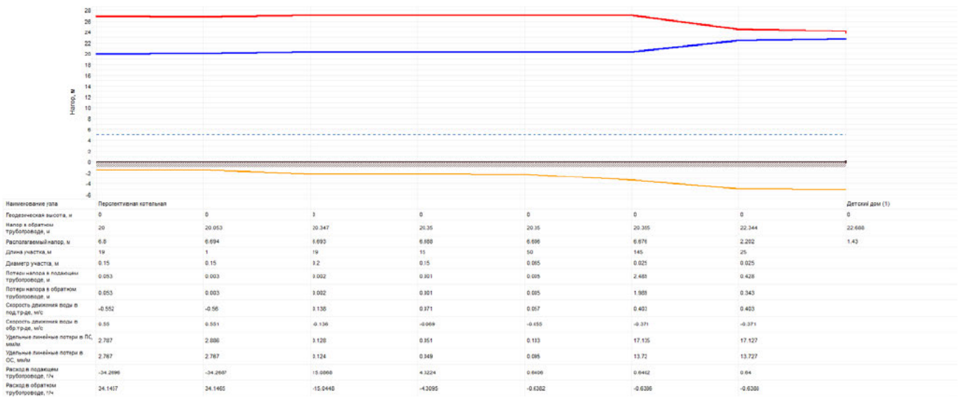
Рисунок 2.9 – Пьезометрический график работы Перспективной котельной
